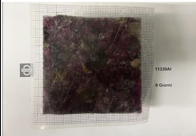
Grado di carbonatazione all'inizio del test
