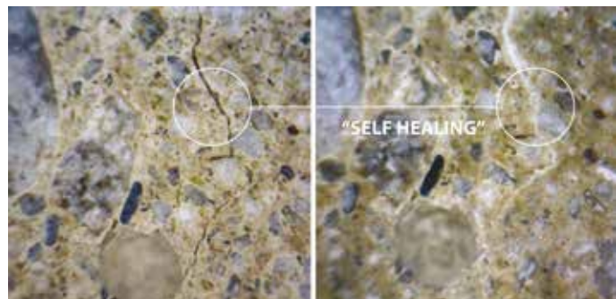
1. L'ingrandimento del fenomeno di autocicatrizzazione "Self Healing" all'interno di una fessurazione
